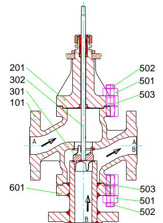
MV 5321, PV 6321 DN 65 – 150, PN 63 – 100
