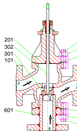
MV 5321, PV 6321 DN 25 – 50, PN 63 – 100
