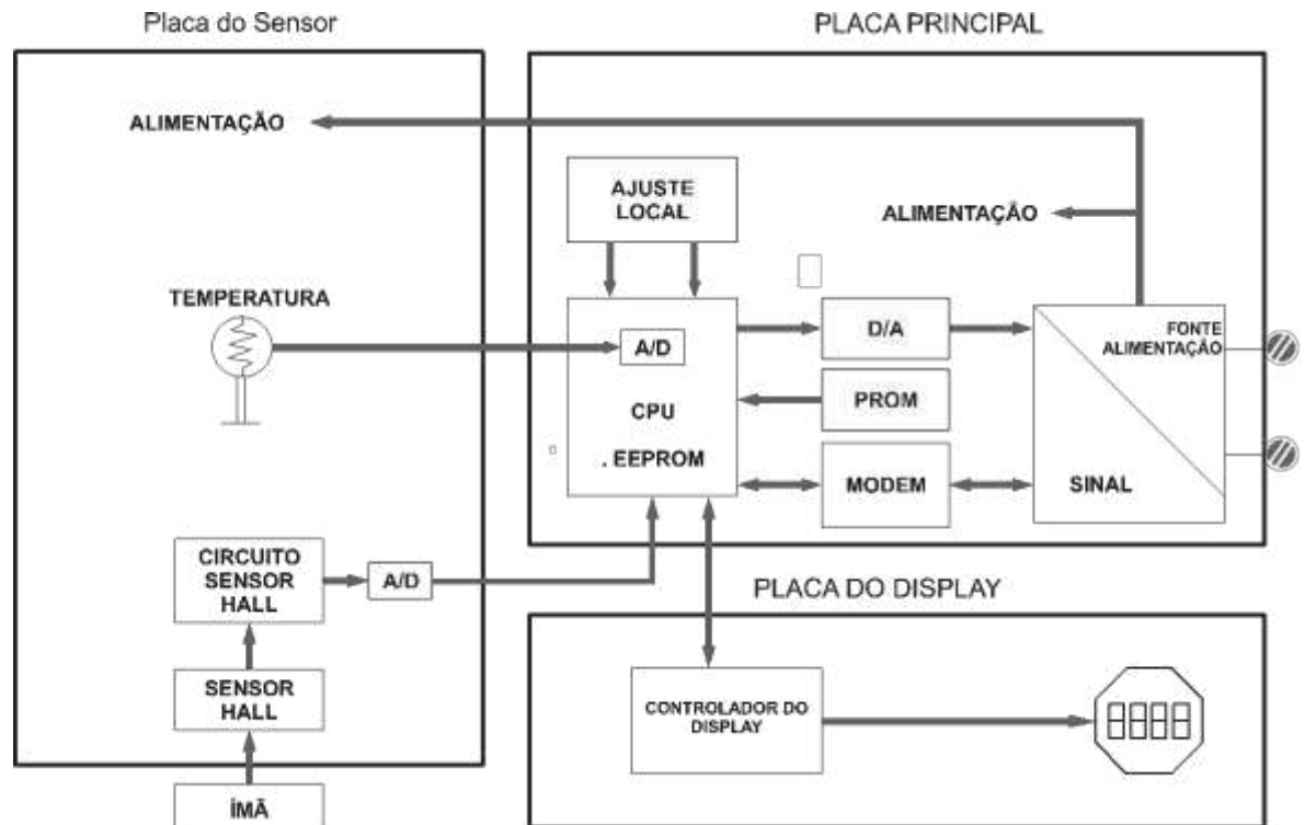
Figura 2.1 – Diagrama de Blocos do TP302
